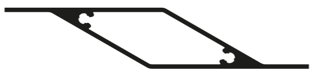
18524 Προφίλ Περισίδας 20x100mm Fence-shade Profile 20x100mm
